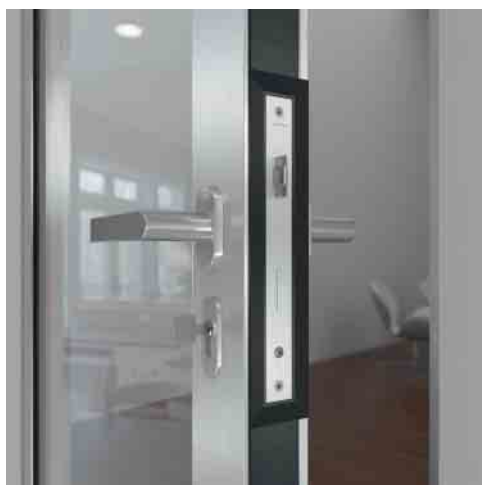
Identischer Türfalzbereich bei Brand- und Rauchschutz Identical door rebate area for fire and smoke protection
